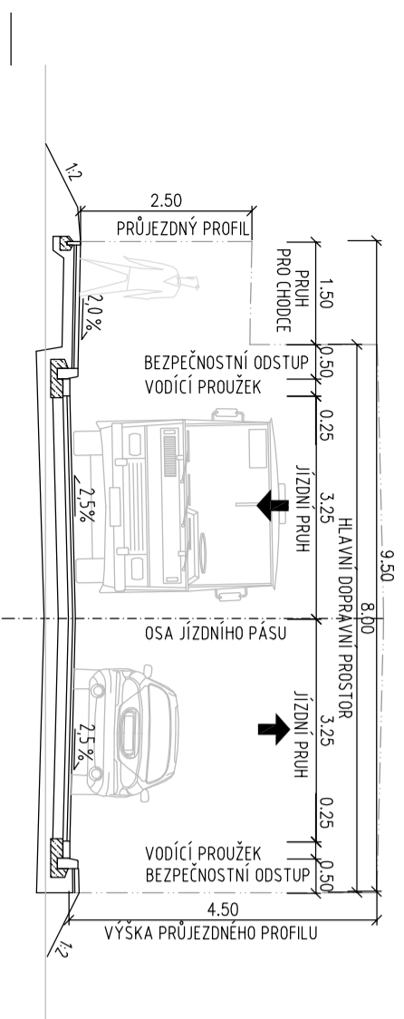
ŘEZ C1 - KM 0,000 MS2 9.5/8.0/40
